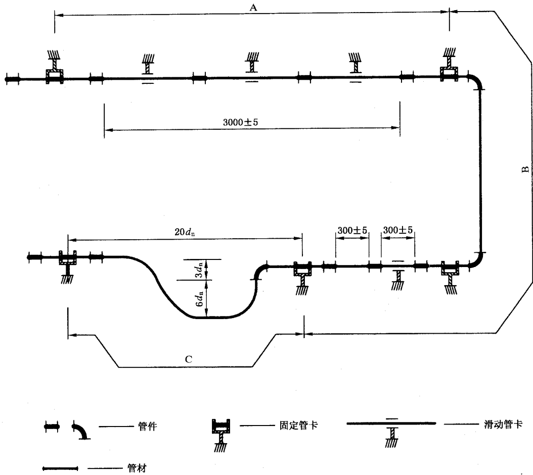
图 A1 试验安装
