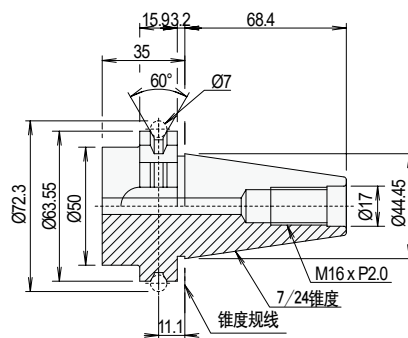
DIN40刀柄
