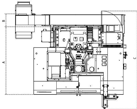
顶视图
