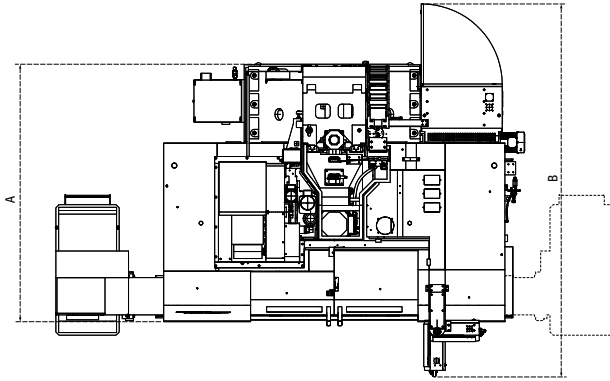
顶视图
