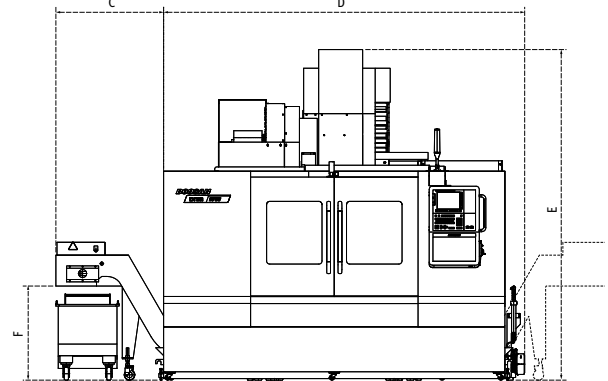
侧视图
