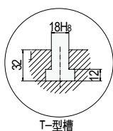
T-型槽
