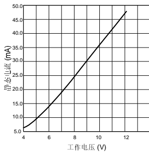
图13 静态电流与工作电压
