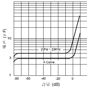
图4 噪声与音量增益设置
