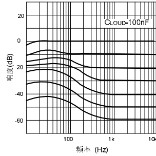
图2 响度、频率与音量衰减
