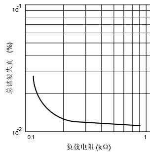
图8 失真与负载电阻
