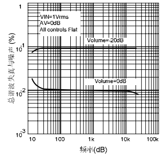
图6 失真、噪声与频率
