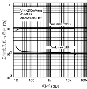
图7 失真、噪声与频率
