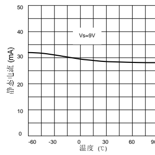
图14 工作电流与温度
