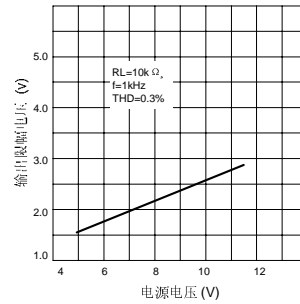
图12 输出限幅电压与电源电压
