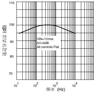
图10 输入分离度(L1, L2, L3, L4) 与频率
