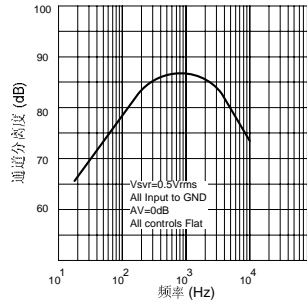
图11 工作电压抑制与频率
