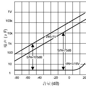
图5 信噪比与音量设置
