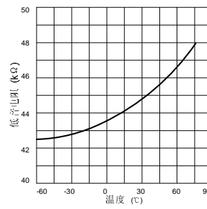
图15 低音提升电阻与温度
