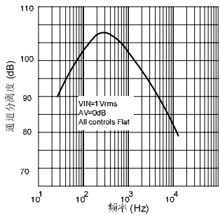
图9 通道分离度(L→R)与频率
