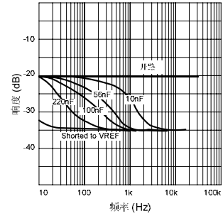
图3 响度与外接电容
