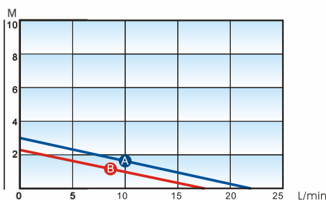
A- 60Hz B- 50Hz 實際輸送液體清水16° C 流量誤差值±10%
