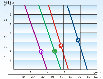
HD-A16: A-7bar B-4bar HD-A6: C-7bar D-4bar
