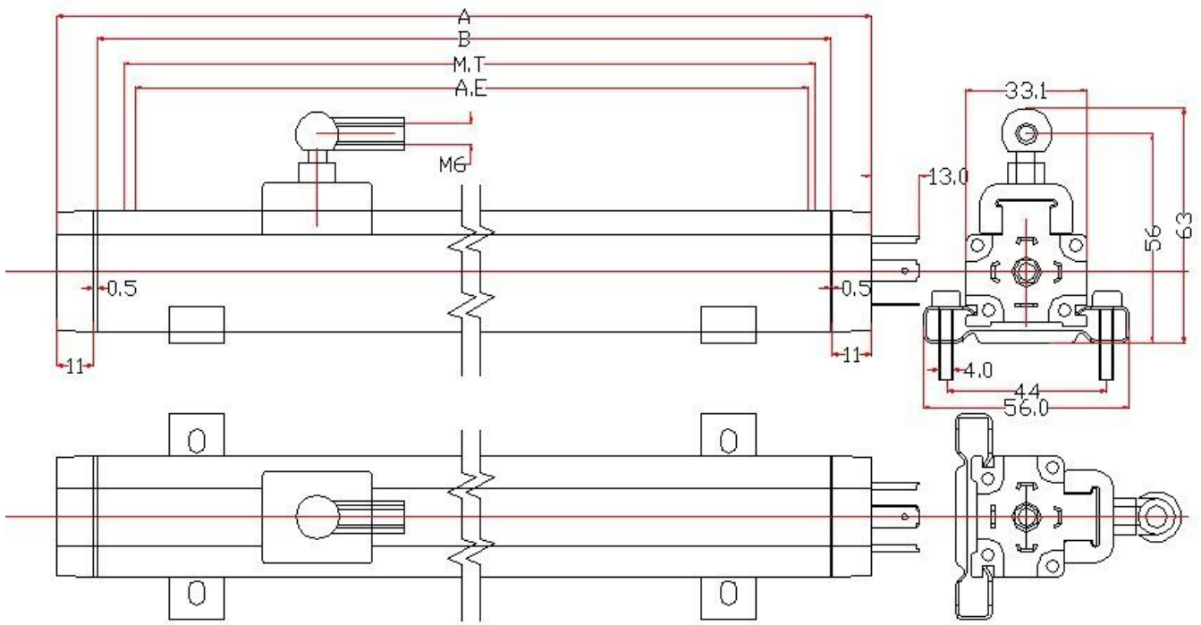
KTF 安装尺寸图
