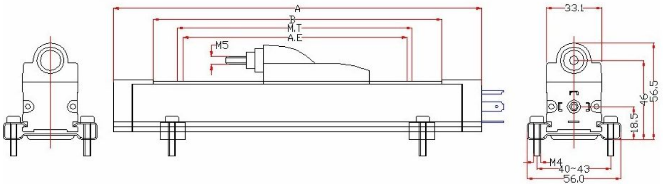
KTF 安装尺寸图
