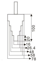
SWRSB1 安全垫块 Safety Block
