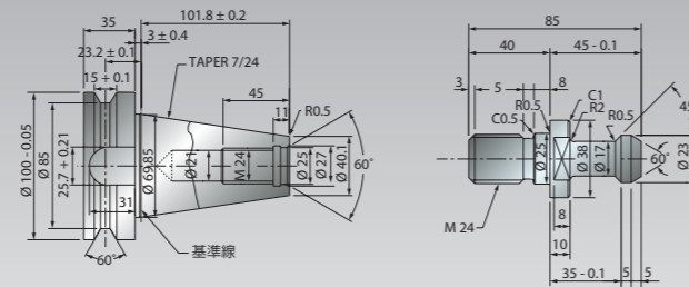
DIN69871-A (#50) (選配)
