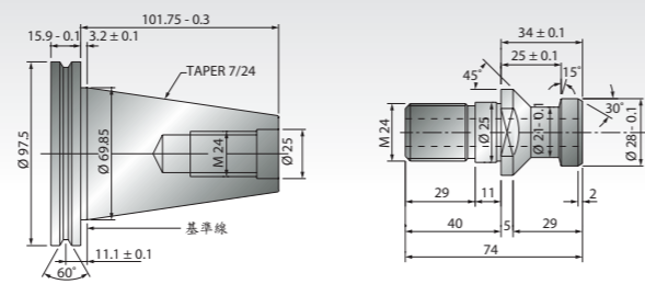
DIN69871-A (#50) (選配)
